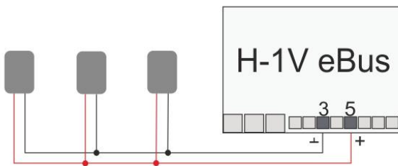
Датчик DS18S20
